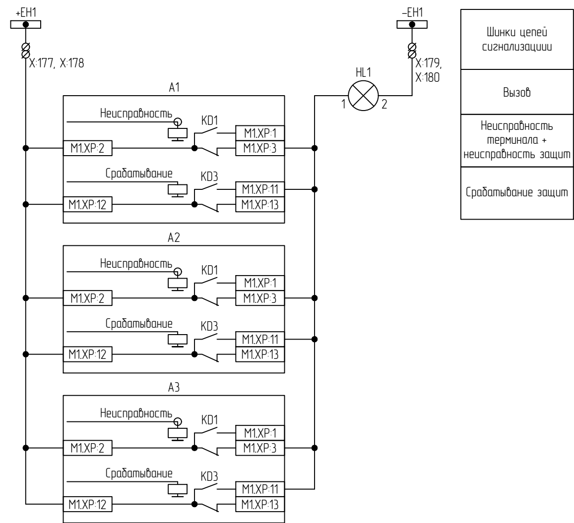
Цепи сигнализации
