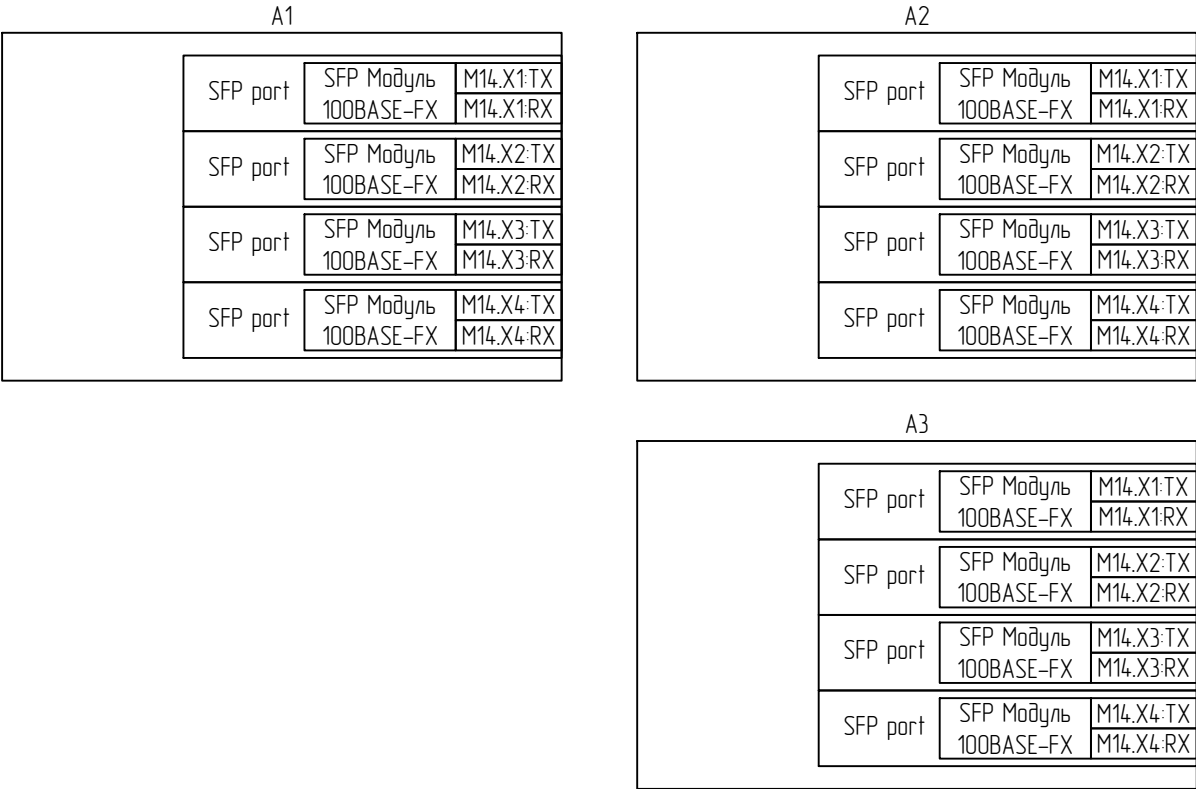
Цепи портов связи терминала
