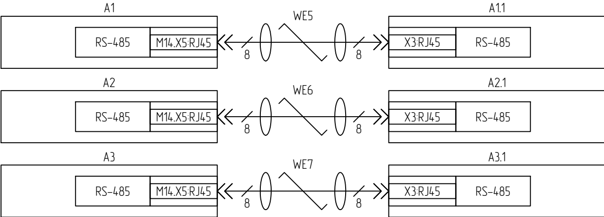
Цепи портов связи терминала
