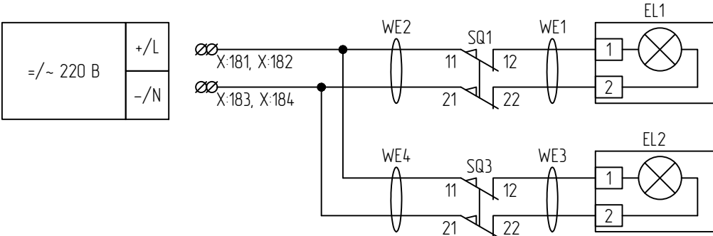
Цепи освещения шкафа
